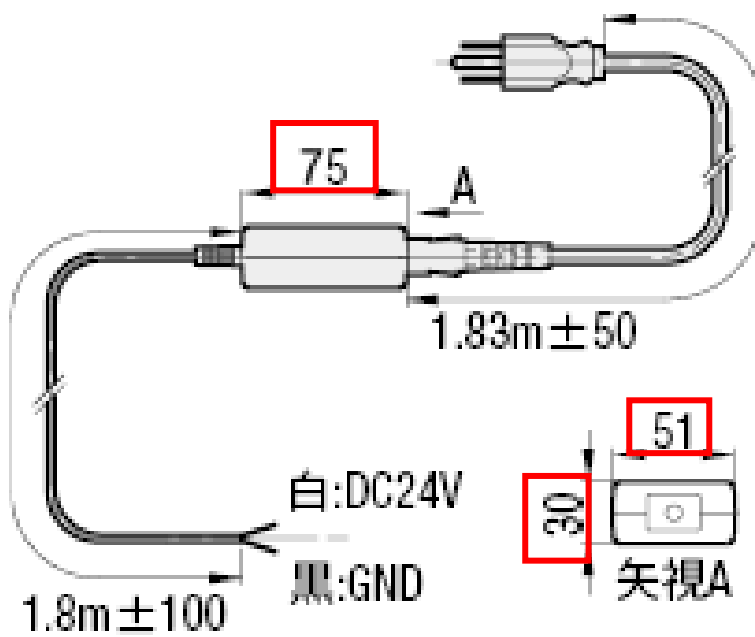
图 2：外形图 修正後
