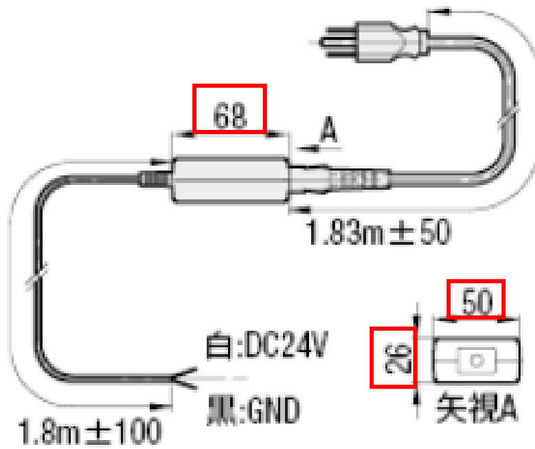
图 1：外形图 修正前
