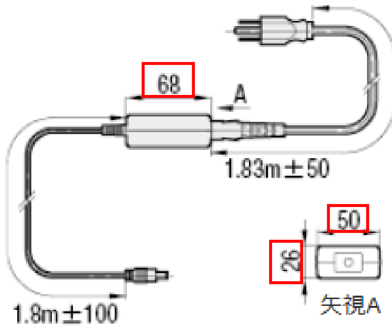
图 1：外形图 修正前
